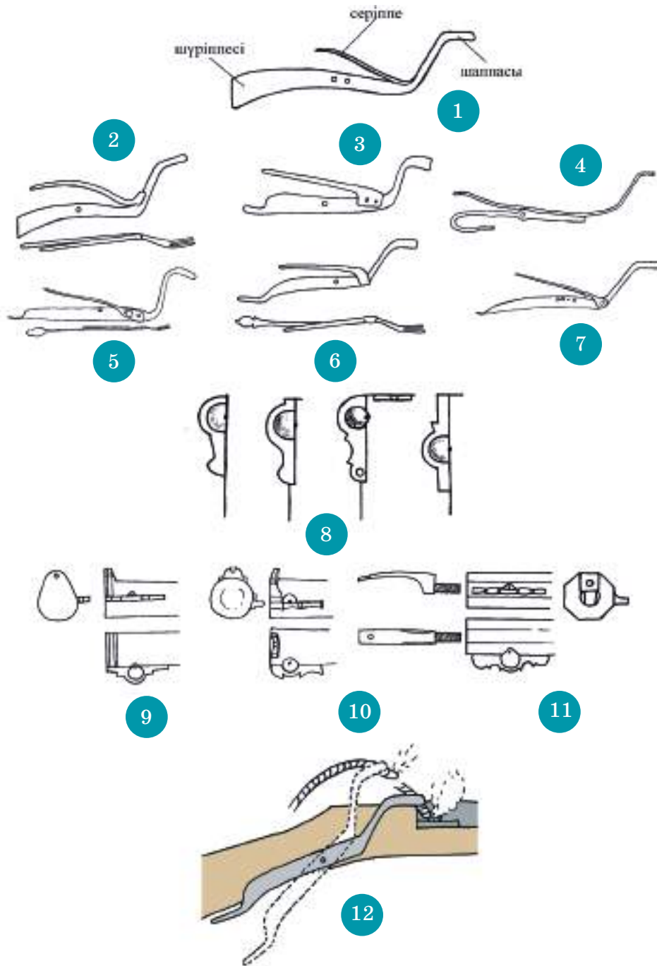
20 - сурет . Пілтелі шүріппе жүйесі. 1-7) Қазақтың пілтелі мылтықтарындағы пілтелік шүріппе түрлері. 8) Оқпанның тұтатқыш дәрі салуға арналған құлақтарының түрлері. 9-11) Пілтелі мылтық оқпанның түбімен бірге соғылған көздеуіші мен түбіне дәнекерленіп бекітілген құлағы. 11) Оқпанның түбіне бұралып бекітілетін теміртегі. ҚР ОММ қорындағы мылтықтардан. XIII-XIX ғғ. 12) Пілтелі шүріппе шаппасына қыстырылған шоқтанған пілтенің оқпан ішіндегі дәріні тұтатуының – пілте мылтықтың атылу әдісінің көрінісі
