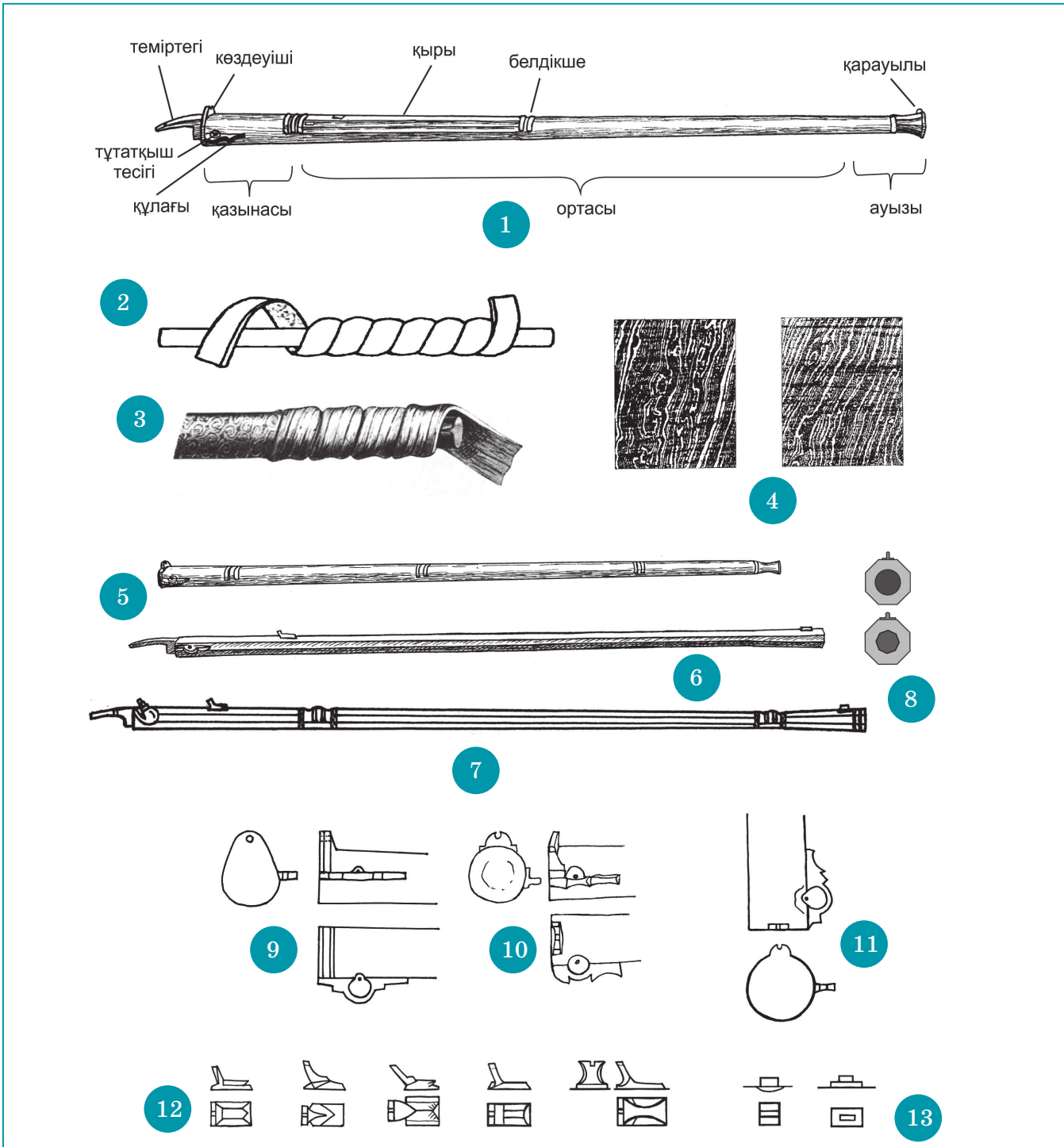
61 сурет. Оқпан. 1) Оқпанның конструктивтік элементтері. 2) Оқпанды болат таспадан орап жасау әдісі. 3) Оқпанды дамашық болаттан орап соғу. 4) Оқпанның дамашық болатының өрнегі. 5-7) Қазақ оқпандарының түрлері. 8) Оқпанның түзу және қырлы ұңғысы. 9-11) Оқпанның түбімен бірге соғылған «шоқтық» түріндегі кездеуіш түрлері. 12) Оқпанның қазына бөлігінің үстінде пазға орнатылатын кездеуіш түрлері. 13) Оқпанның қарауылы
