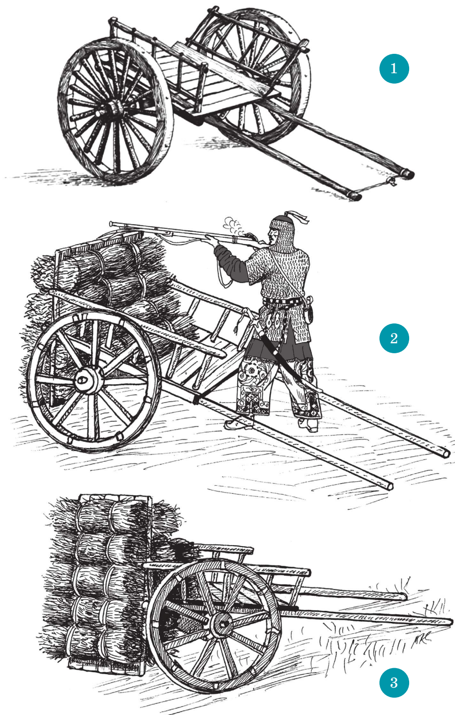
77-сурет. Қазақтың жылжымалы мантелеті – қамыстан, шөптен, бұталардан жіппен буылып жасаған байламаларды қалқан қылып орнатқан екі дөңгелекті арба. 1) Қазақтың екі дөңгелекті арбасы. Ж. Шайкеннің суреті. 2, 3) Қазақ мантелетінің алды-артынан көрінісі және оның тасасымен атыс жүргізу әдісі. Жазба деректер бойынша автордың қалпына келтірген суреті
