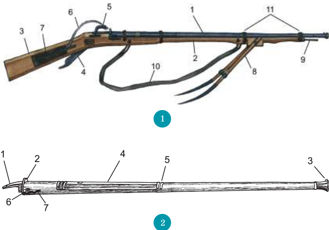
17-сурет. Қолға ұстап ататын отты қару – мылтық.
