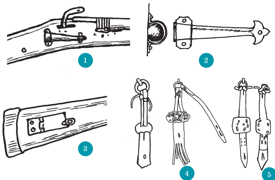
60 - сурет . Қазақ мылтықтарының дүміне орнатылған, мылтықты күтуге, жөндеуге қажетті ұсақ саймандарды сақтауға арналған сауыт, қалталар
