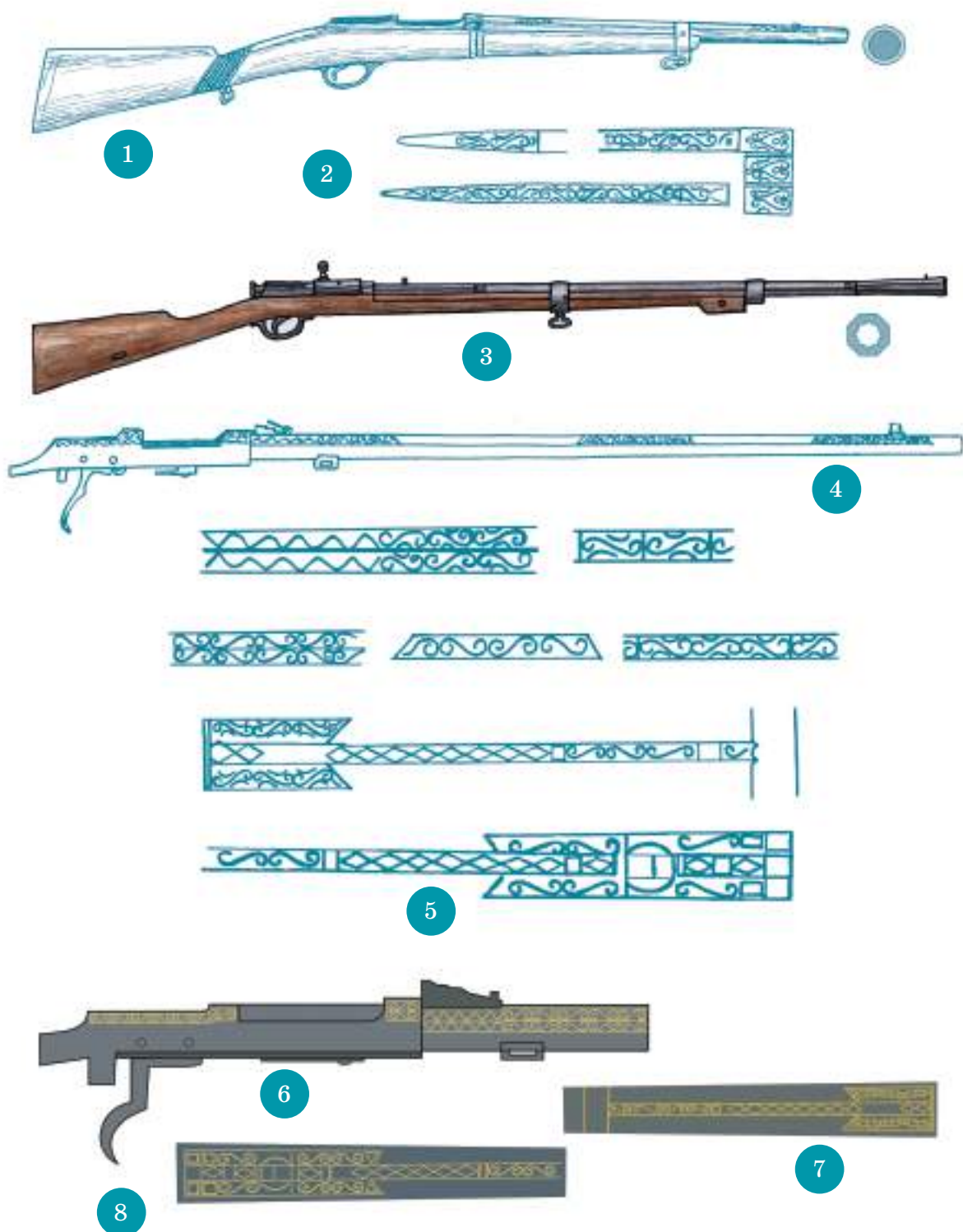
38 сурет. Бердеңке мылтық. 1, 3) Қазақтың бердеңке мылтықтары. XIX ғ. аяғы. ҚР ОММ қорынан. 4) Қазақ бердеңке мылтығының оқпаны. XIX ғ. аяғы – XX ғ. басы. ҚР ОММ қорынан. 2, 5-8) Оқпанды әшекейлеуде қолданылған ою-өрнектер.
